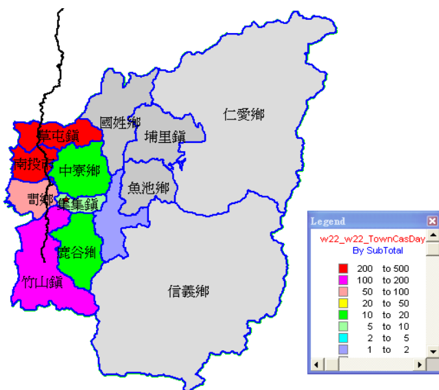
圖五-3 模擬車籠埔斷層白天人員傷亡分布圖
