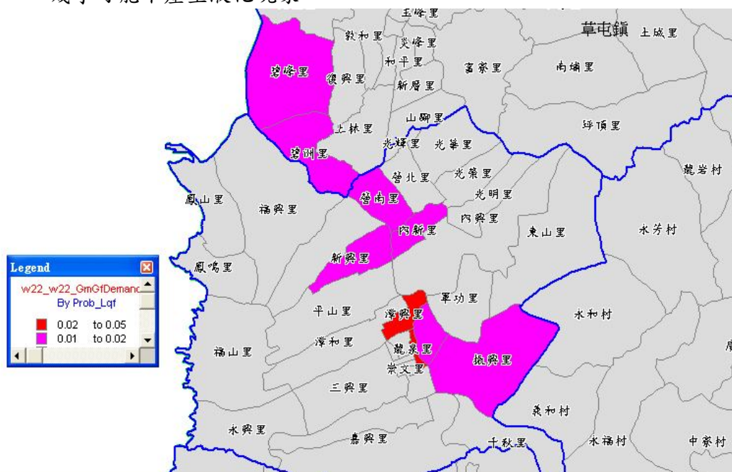
圖五-5 模擬車籠埔斷層對南投縣境內液化之機率
