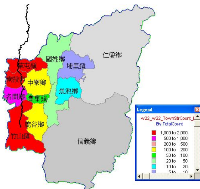
圖五-2 模擬車籠埔斷層建物至少嚴重損毀分布圖
