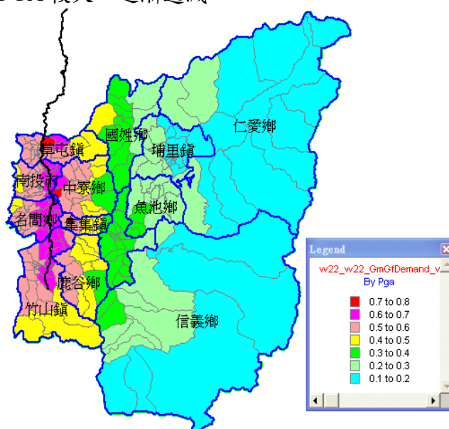
圖五-1 模擬車籠埔斷層 PGA 分布圖
